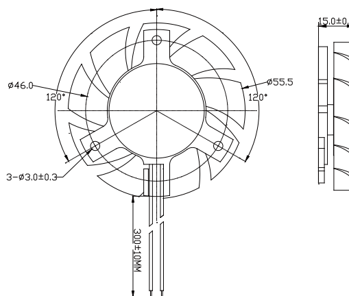
尺寸图 / Dimension drawing
