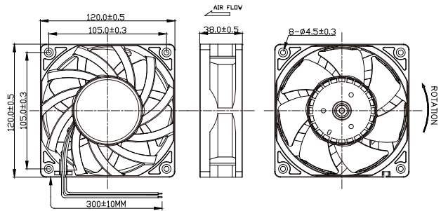
尺寸图 / Dimension drawing
