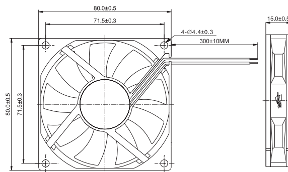
尺寸图 / Dimension drawing
