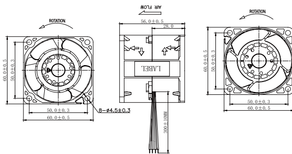
尺寸图 / Dimension drawing
