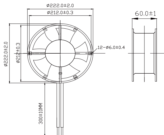
尺寸图 / Dimension drawing
