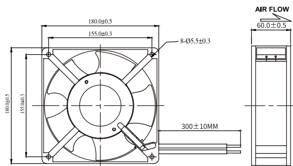
尺寸图 / Dimension drawing
