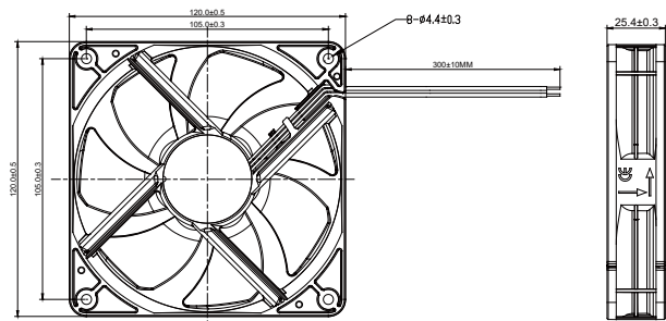
尺寸图 / DIMENSIONS DRAWING
